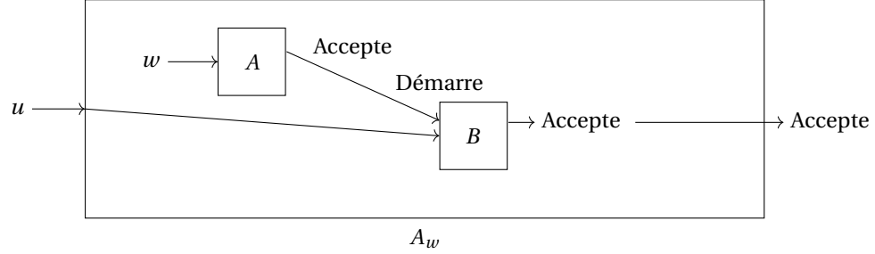
FIGURE 9.10 – Illustration de la machine de Turing utilisée dans la preuve du théorème de Rice.
