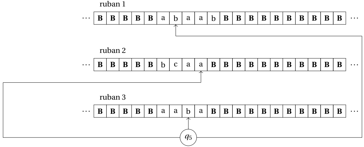
FIGURE 7.3 – Une machine de Turing à 3 rubans
