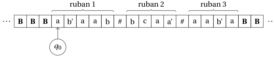
FIGURE 7.4 – Illustration de la preuve de la proposition 7.22 : représentation graphique d’une machine de Turing à 1 ruban simulant la machine à 3 rubans de la figure 7.3. Sur cette représentation graphique, on écrit une lettre primée lorsque le bit “la tête de lecture est en face de cette case” est à 1.
