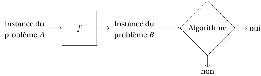
FIGURE 9.6 – Réduction du problème A vers le problème B . Si l'on peut résoudre le problème B , alors on peut résoudre le problème A . Le problème A est donc plus facile que le problème B , noté A \leq_m B .
