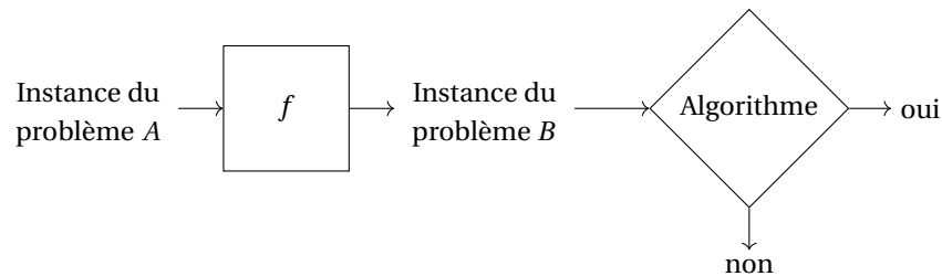
FIGURE 12.1 – Les réductions transforment des instances positives en instances positives, et négatives en négatives.
