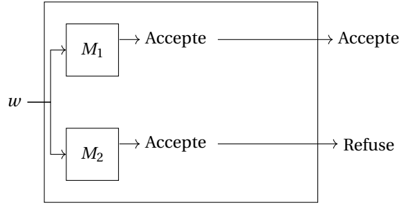
FIGURE 9.3 – Illustration de la preuve du théorème 9.24.
