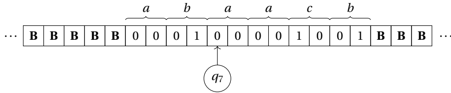
FIGURE 7.2 – Illustration de la preuve de la proposition 7.21.
