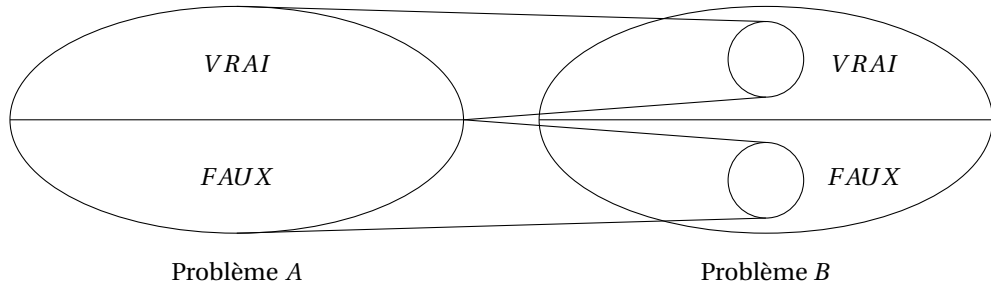
FIGURE 9.7 – Les réductions transforment des instances positives en instances positives, et négatives en négatives.
