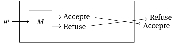
FIGURE 9.4 – Construction d’une machine de Turing acceptant le complément d’un langage décidable.
