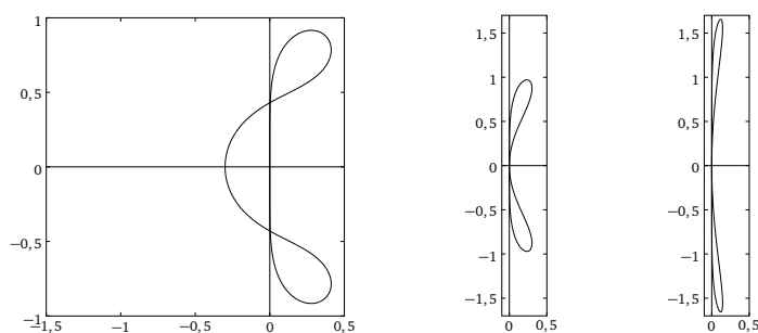
FIGURE 8.17 – Courbes du lieu des racines des méthodes d'Adams–Bashforth à quatre pas (à gauche), de Nystrom à trois pas (au milieu) et de Milne–Simpson généralisée à quatre pas (à droite).
