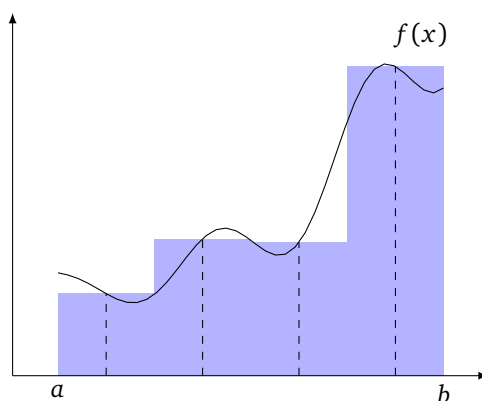
FIGURE 7.4 – Illustration de la règle du point milieu composée à quatre sous-intervalles sur l'intervalle [a, b] . La valeur approchée I_{4,0}(f; a, b) de l'intégrale I(f; a, b) correspond à l'aire colorée en bleu.
