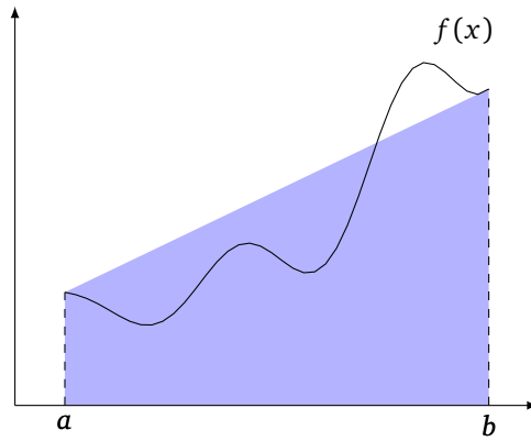
FIGURE 7.2 – Illustration de la règle du trapèze. La valeur approchée I_1(f; a, b) de l'intégrale I(f; a, b) correspond à l'aire colorée en bleu.
