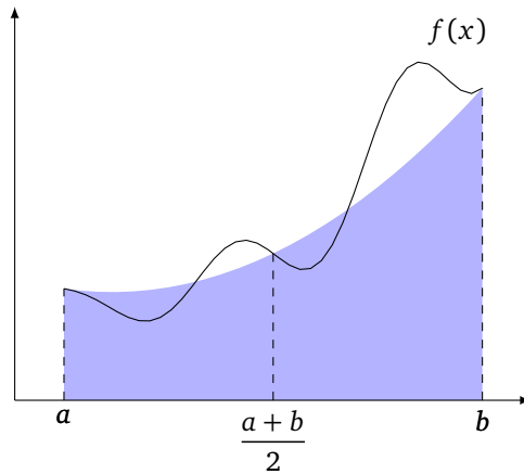
FIGURE 7.3 – Illustration de la règle de Simpson. La valeur approchée I_2(f; a, b) de l'intégrale I(f; a, b) correspond à l'aire colorée en bleu.
