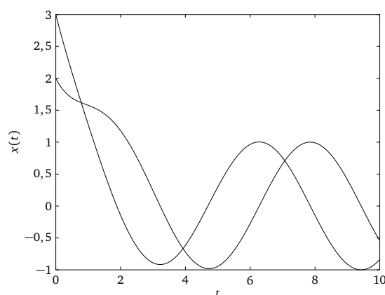
FIGURE 8.23 – Solution des problèmes (8.113) et (8.114) sur l'intervalle [0, 10] .
