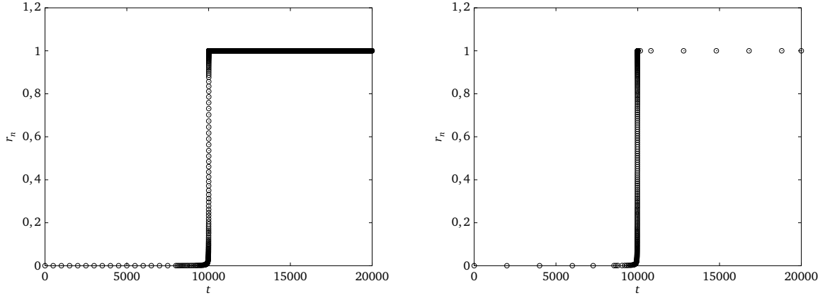
FIGURE 8.22 – Solutions numériques approchées du problème (8.112) sur l'intervalle [0, \frac{2}{\delta}] , pour \delta = 10^{-4} , respectivement obtenues par une méthode de Runge-Kutta emboîtée (à gauche) et une méthode de Rosenbrock modifiée (à droite), combinées à une stratégie d'adaptation du pas de discrétisation.
