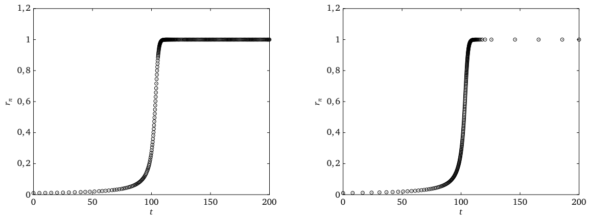
FIGURE 8.21 – Solutions numériques approchées du problème (8.112) sur l'intervalle [0, \frac{2}{\delta}] , pour \delta = 10^{-2} , respectivement obtenues par une méthode de Runge–Kutta emboîtée (à gauche) et une méthode de Rosenbrock modifiée (à droite), combinées à une stratégie d'adaptation du pas de discrétisation.
