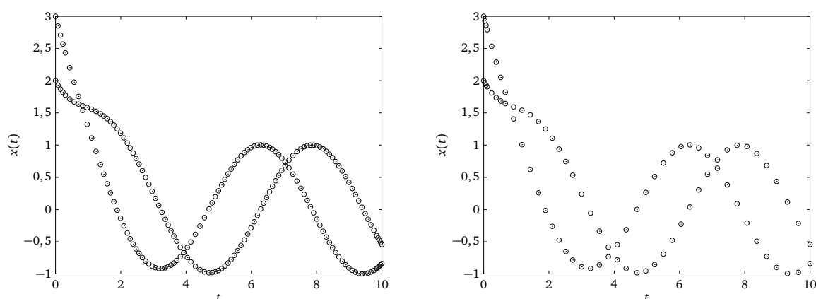
FIGURE 8.24 – Solutions numériques approchées du problème (8.113) sur l'intervalle [0, 10] respectivement obtenues par une méthode de Runge-Kutta emboîtée (à gauche) et une méthode de Rosenbrock modifiée (à droite), combinées à une stratégie d'adaptation du pas de discrétisation.
