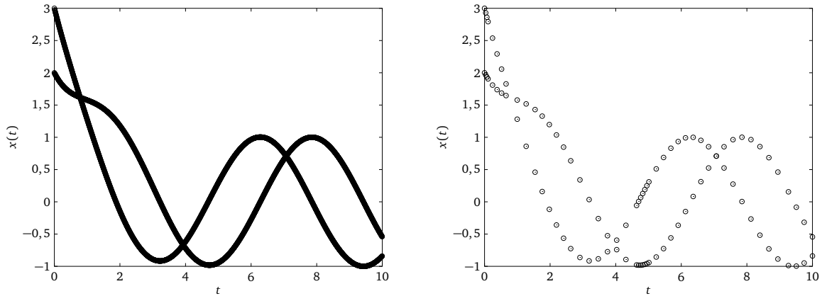
FIGURE 8.25 – Solutions numériques approchées du problème (8.114) sur l'intervalle [0, 10] respectivement obtenues par une méthode de Runge–Kutta emboîtée (à gauche) et une méthode de Rosenbrock modifiée (à droite), combinées à une stratégie d'adaptation du pas de discrétisation..
